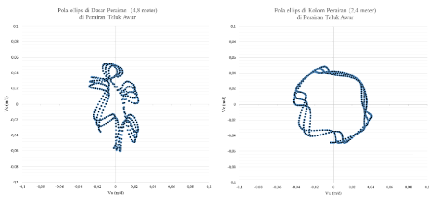
Pola ellips Arus Harmonik di Dasar Perairan
