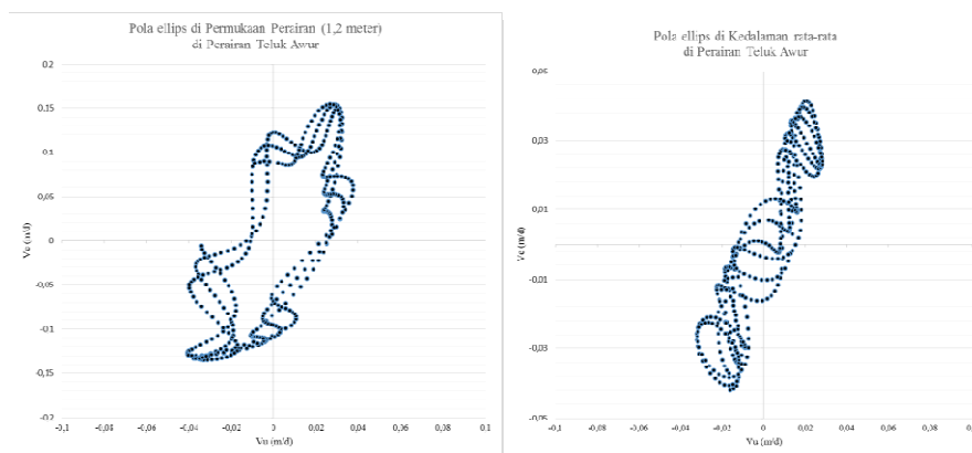
Gambar 3. Pola ellips Arus Harmonik di Permukaan Perairan
