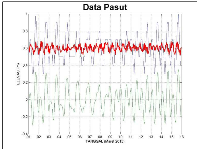
Gambar 5. Grafik Pola Pasang Surut Harmonik dan Pola Arus Admiralty (keterangan: elevasi harmonik(warna merah); elevasi admiralty (warna biru); elevasi residu (warna hijau))
