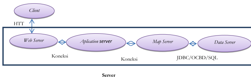
Gambar 2. Arsitektur Multi-tier generic Client-server Web GIS (diadopsi dari Rao, 2010)
